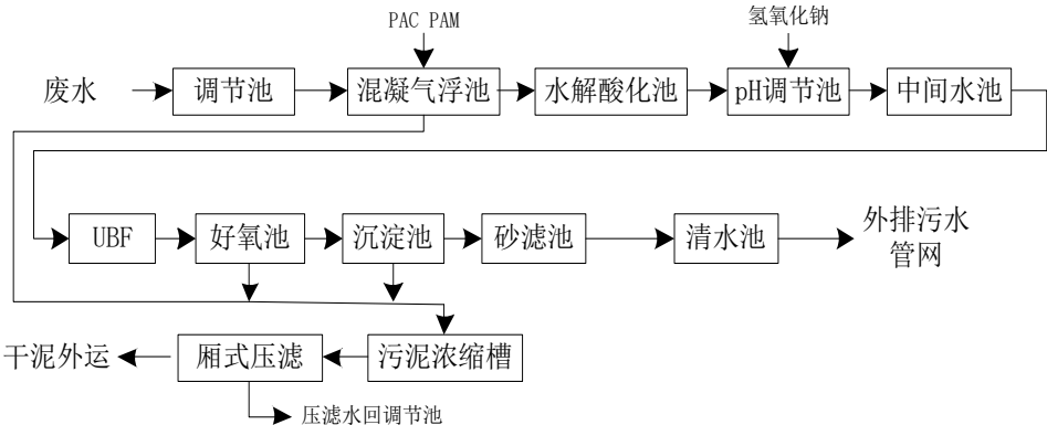
图 4-2 比亚迪污水处理站工艺流程
