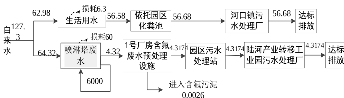
图 2-1 本项目水平衡图 (m³/d)
